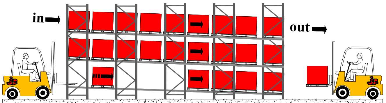
Front view Hình mặt trước
