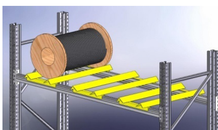
For cable axis Đặt trụ gỗ dây cáp điện
