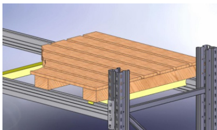
For pallet Đặt Ba lét
