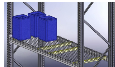
With wire mesh for loose cargo Lót tấm lưới để trữ hàng
