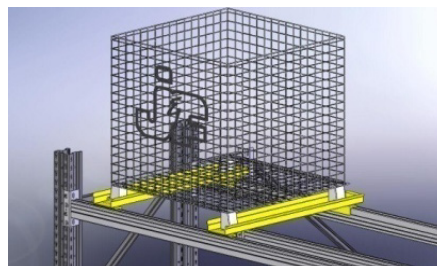
For wire mesh container Đặt lồng trữ hàng
